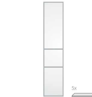
VESTA 1650 mm, L,R HSV 1650 0350.5 - vestavný model, 3 dvířka, L HSV 1650 0350.6 - vestavný model, 3 dvířka, R
