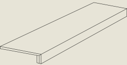
SCALINO INCOLLATO GLUED STEP TREAD / NEZ DE MARCHE COLLÉ / GEKLEBTE STUFENPLATTE / PELDAÑO CON PERFIL PEGADO ■ 33x120 (13"x48") RT 9mm
