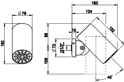
57203 Hlavová sprcha pro instalaci na stěnu. Polohovatelná. Funkce: déšť. Pozn.: všechny hlavové sprchy Spotwater můžou být použity na sprchovém sloupu.
